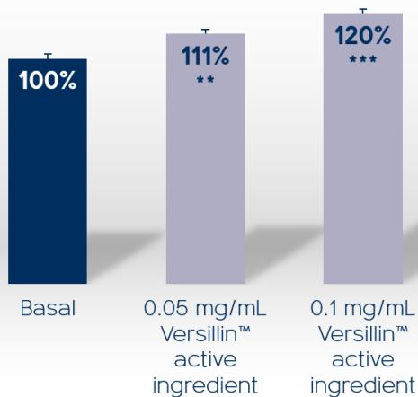
Синтез тропоэластина (%)
